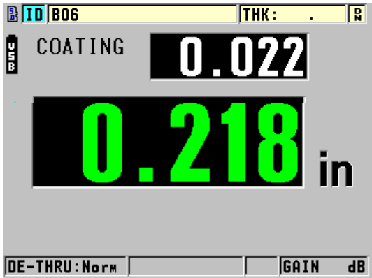
Medición THRU-COAT que muestra el espesor del revestimiento y del acero (A-scan no activo)
