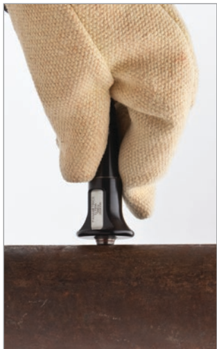
Palpador (o sonda) D790-SM sobre tubo, bajo condiciones de alta temperatura
